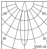
2117.433-V
