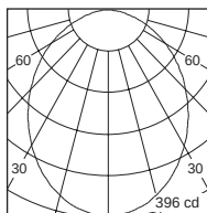
2117.420A-V
